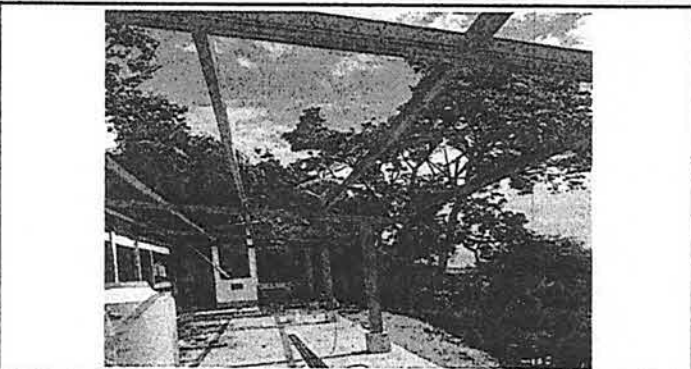
FOTO 5: INSTALACIÓN DE ESTRUCTURA DE METAL PARA SOPORTE DE LÁMINA
